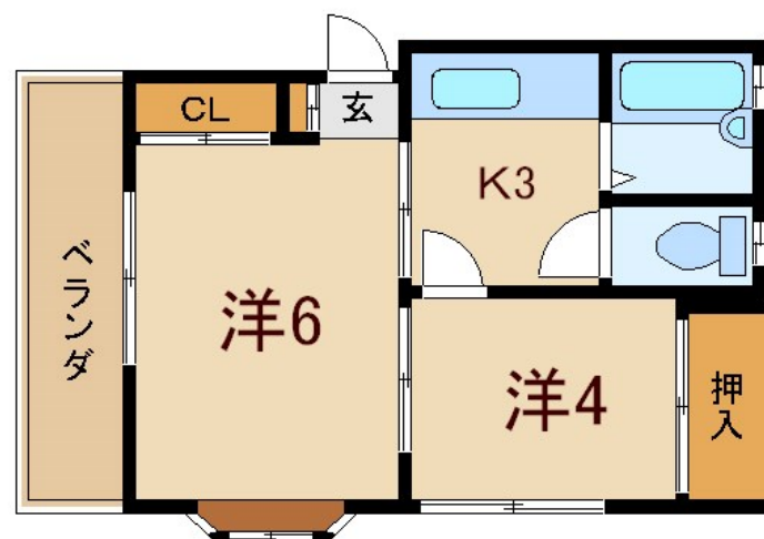
【間取り図】
