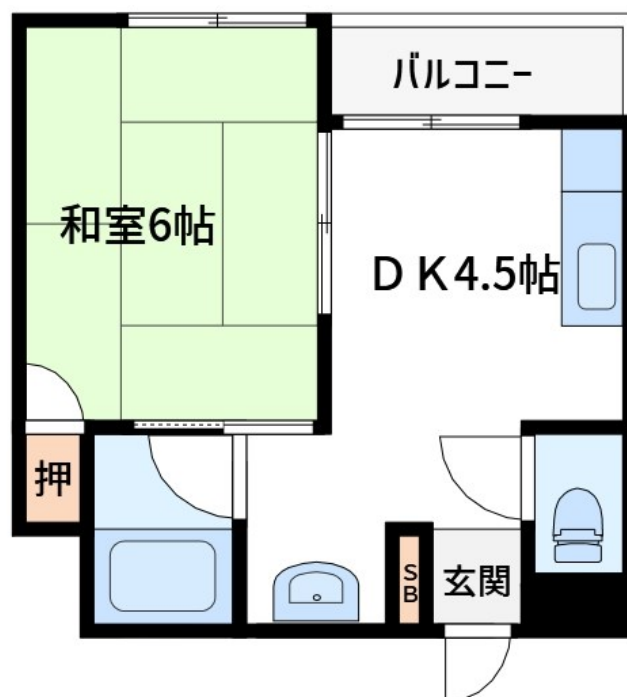
【間取り図】
