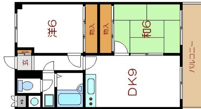
【間取り図】
