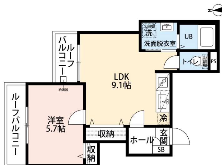
【間取り図】
