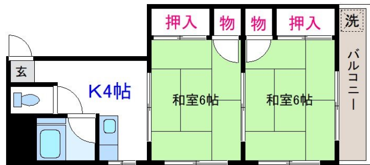
【間取り図】
