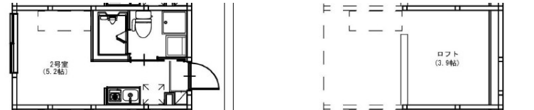
【間取り図】
