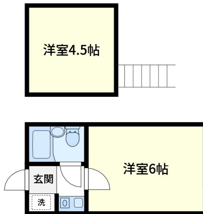
【間取り図】
