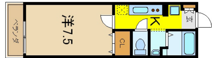
【間取り図】
