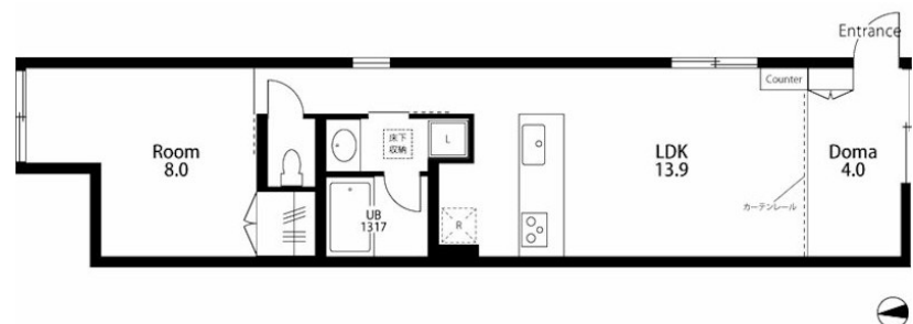
【間取り図】
