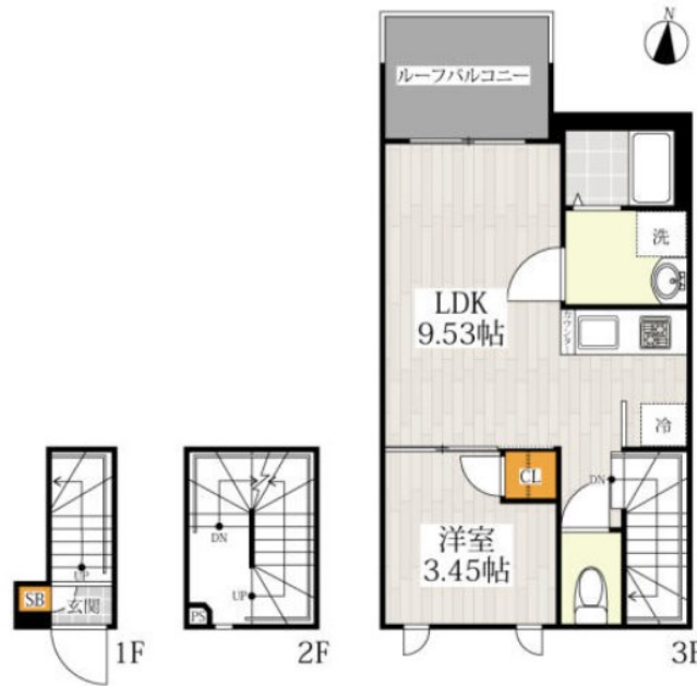
【間取り図】
