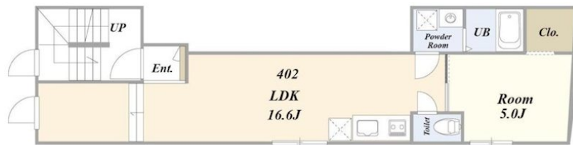
【間取り図】
